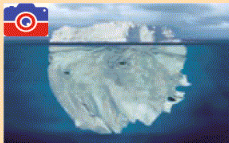
Fig. 1. Aisberg
