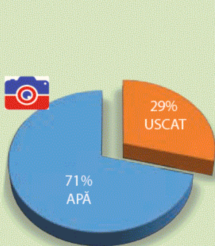
Fig. 1. Diagrama proporției uscat-apă
