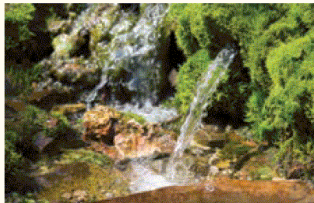
Fig. 3. Izvor
