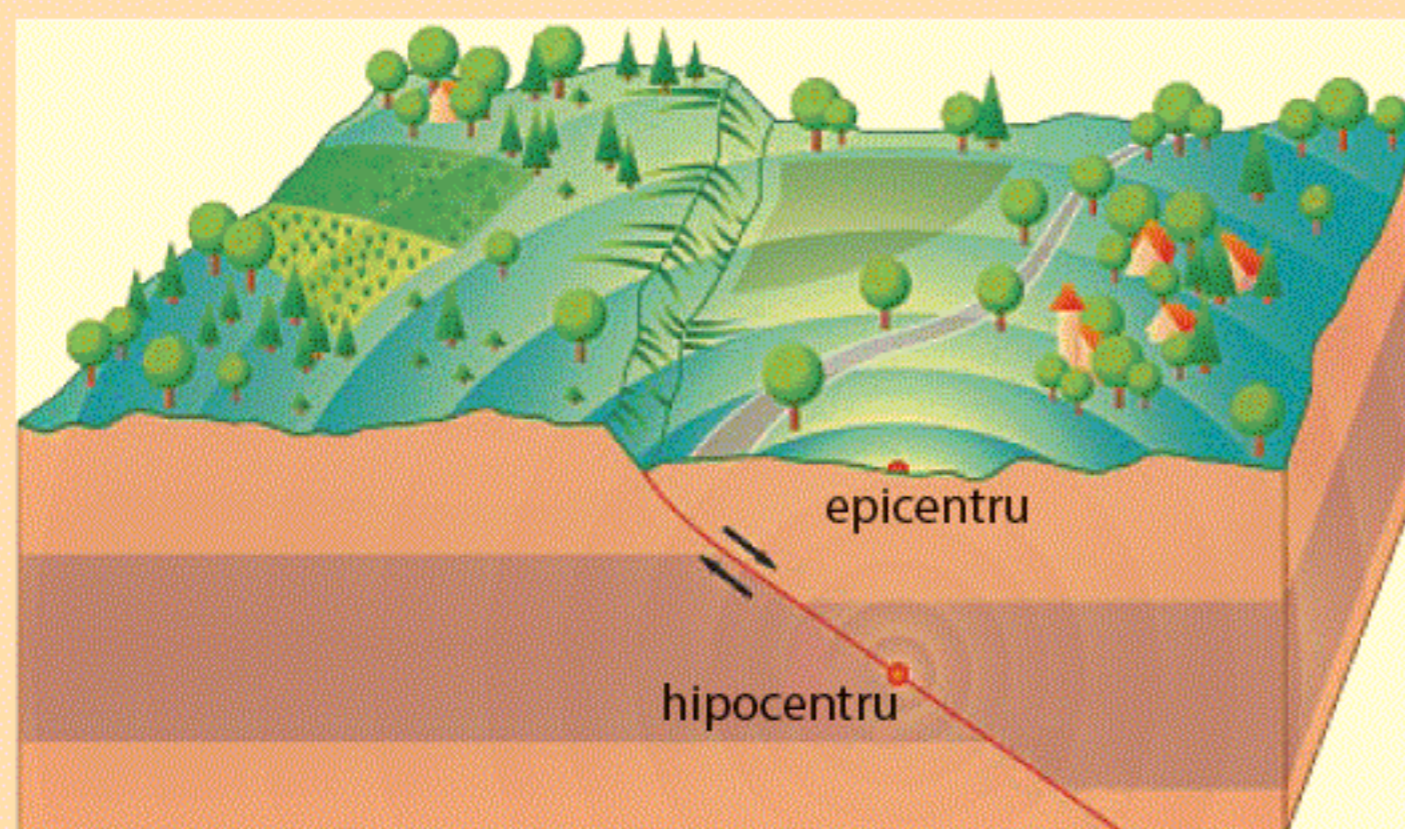
Fig. 4. Producerea unui cutremur
