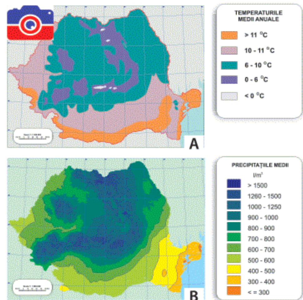
Fig. 1. Harta temperaturilor medii anuale (A); harta precipitațiilor medii anuale (B)
