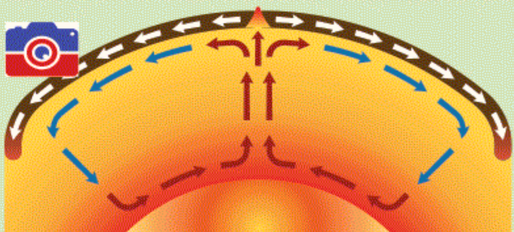
Fig. 3. Curenți în magmă
