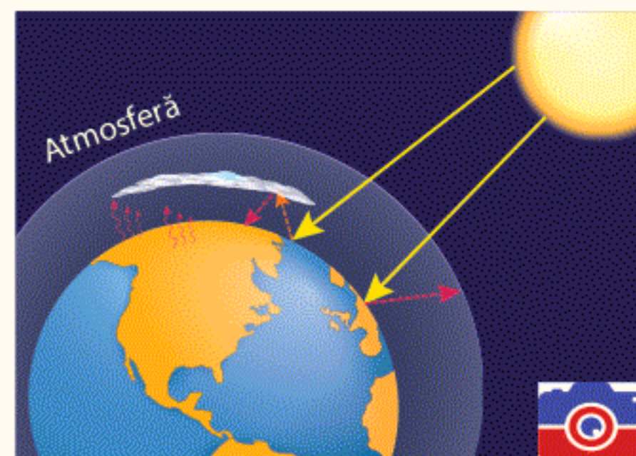
Fig. 1. Încălzirea atmosferei
