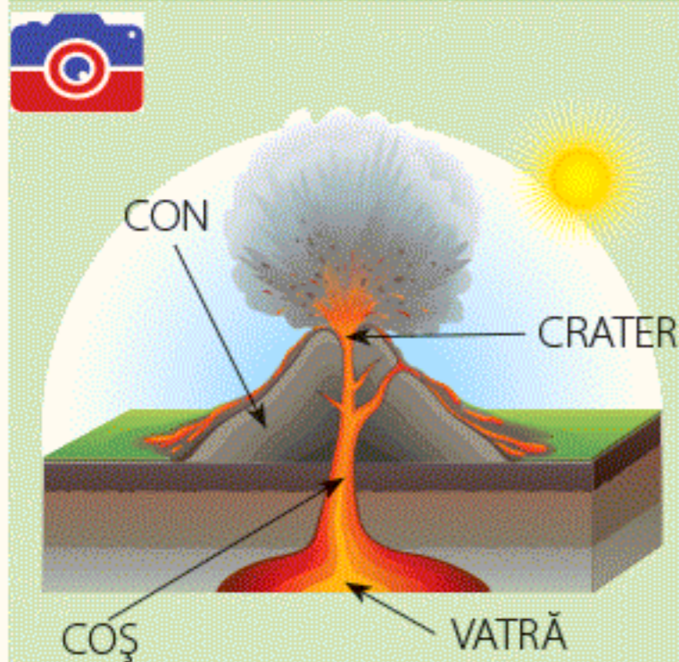
Fig. 2. Părțile componente ale unui vulcan
