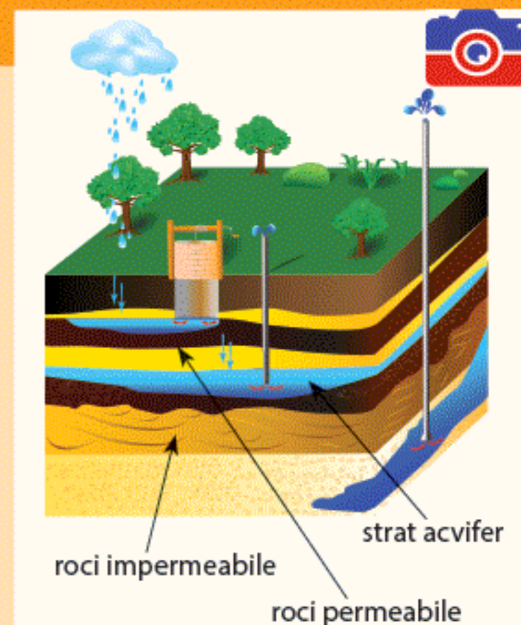
Fig. 1. Formarea stratului acvifer
