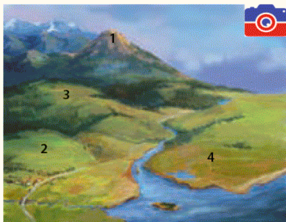
Fig. 3. Forme de relief
