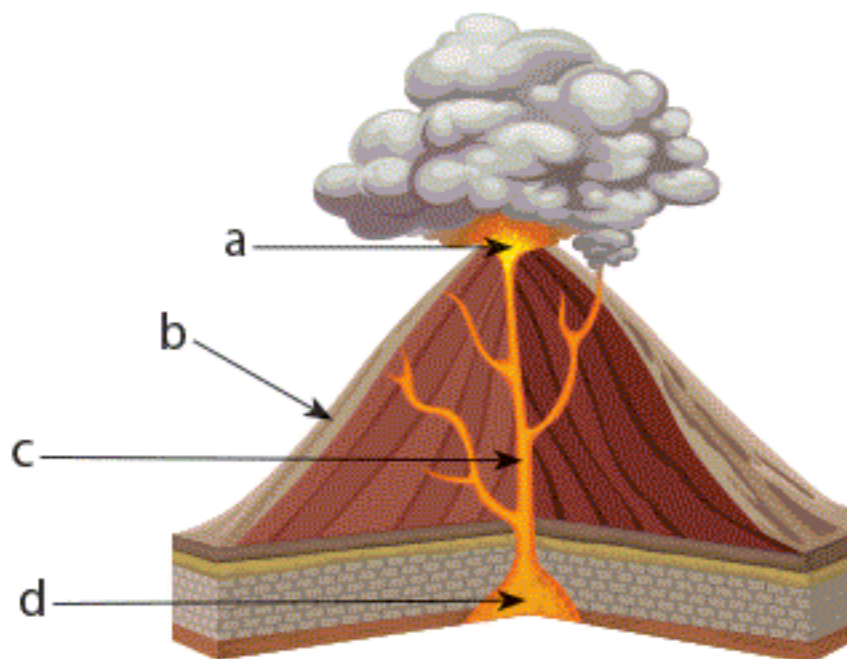
Fig. 2. Secțiune într-un vulcan
