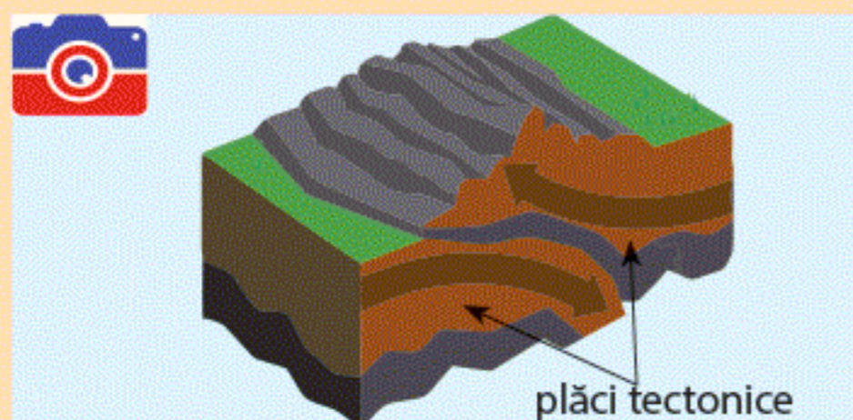
Fig. 4. Formarea munților de încrețire
