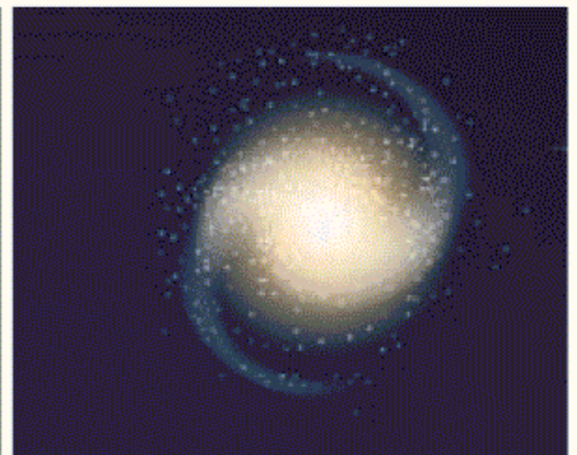
Fig. 3. Galaxie spiralată
