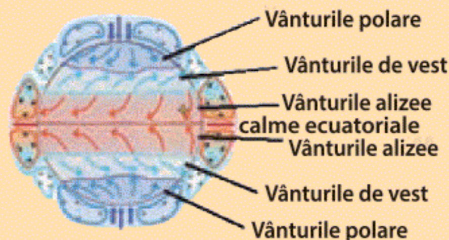
Fig. 4. Vânturile permanente
