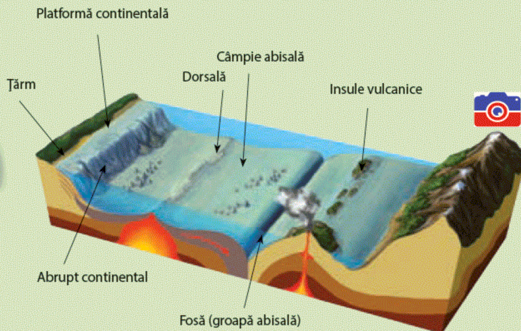
Fig. 2. Formele de relief ale bazinelor oceanice
