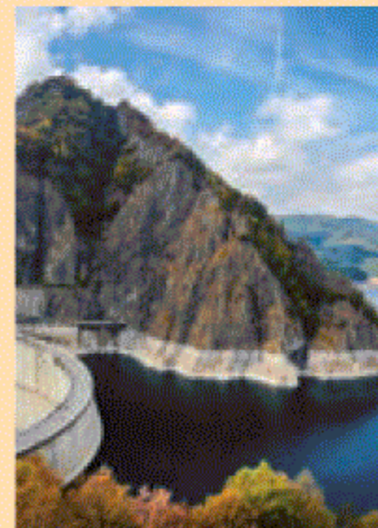
Fig. 5. Lacul Vidraru
