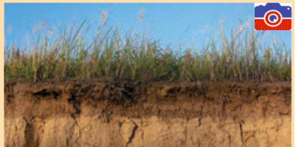
Fig. 3. Sol
