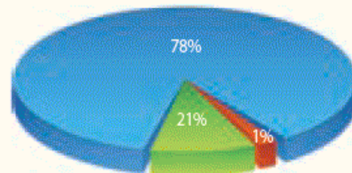
Fig. 1. Proporția gazelor din compoziția atmosferei
