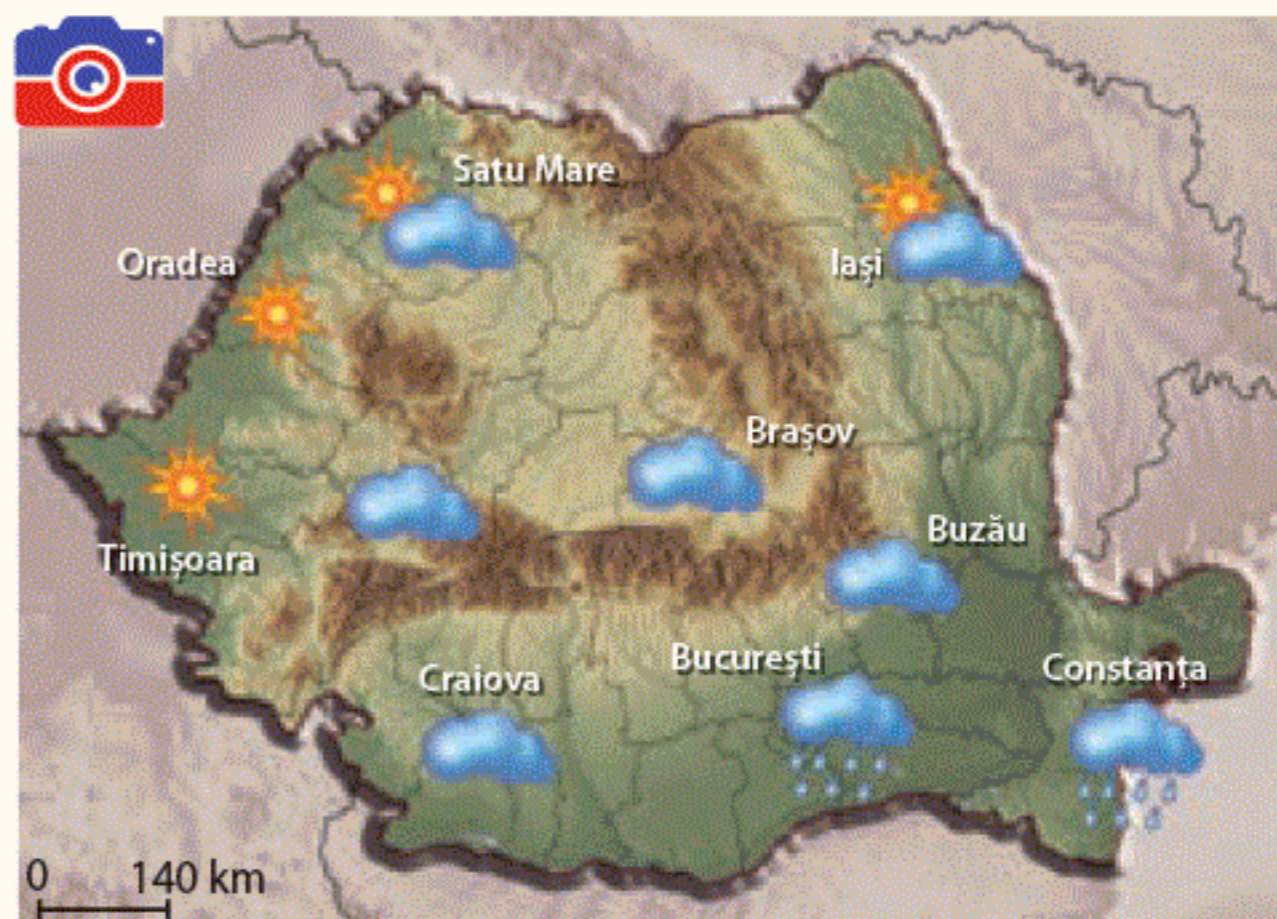
Fig. 2. Hartă meteorologică
