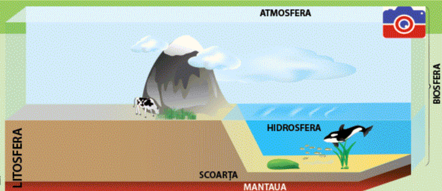
Fig. 1. Învelișurile Pământului
