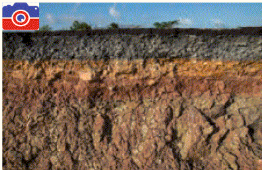
Fig. 2. Straturi de roci permeabile
