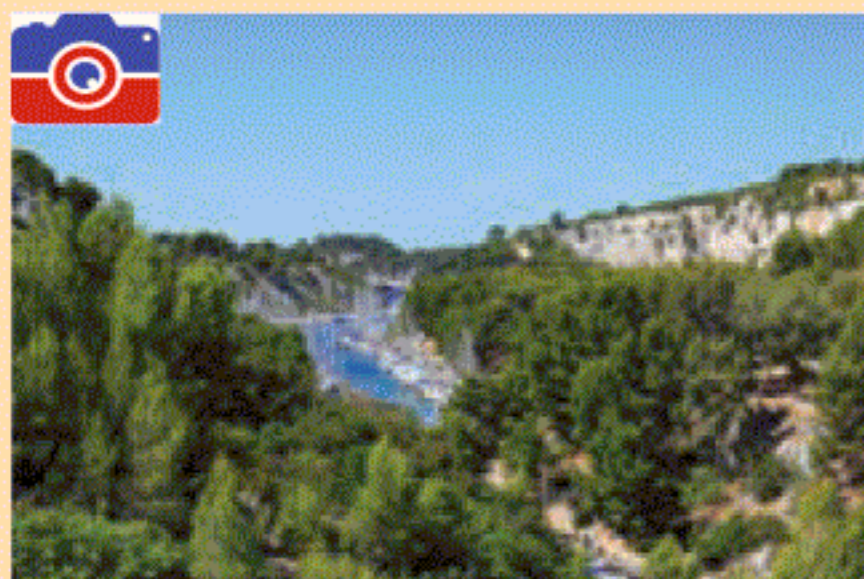
Fig. 6. Peisaj mediteraneeen
