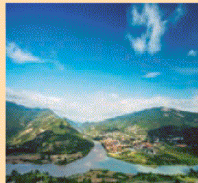
Fig. 6. Confluență
