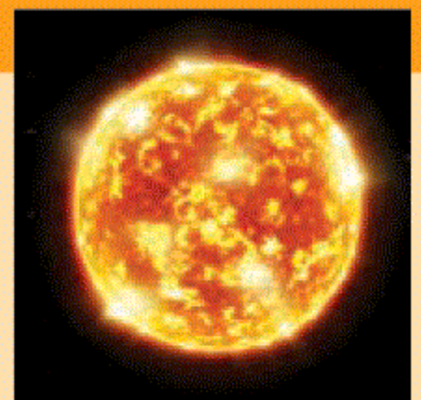
Fig. 2. Soarele
