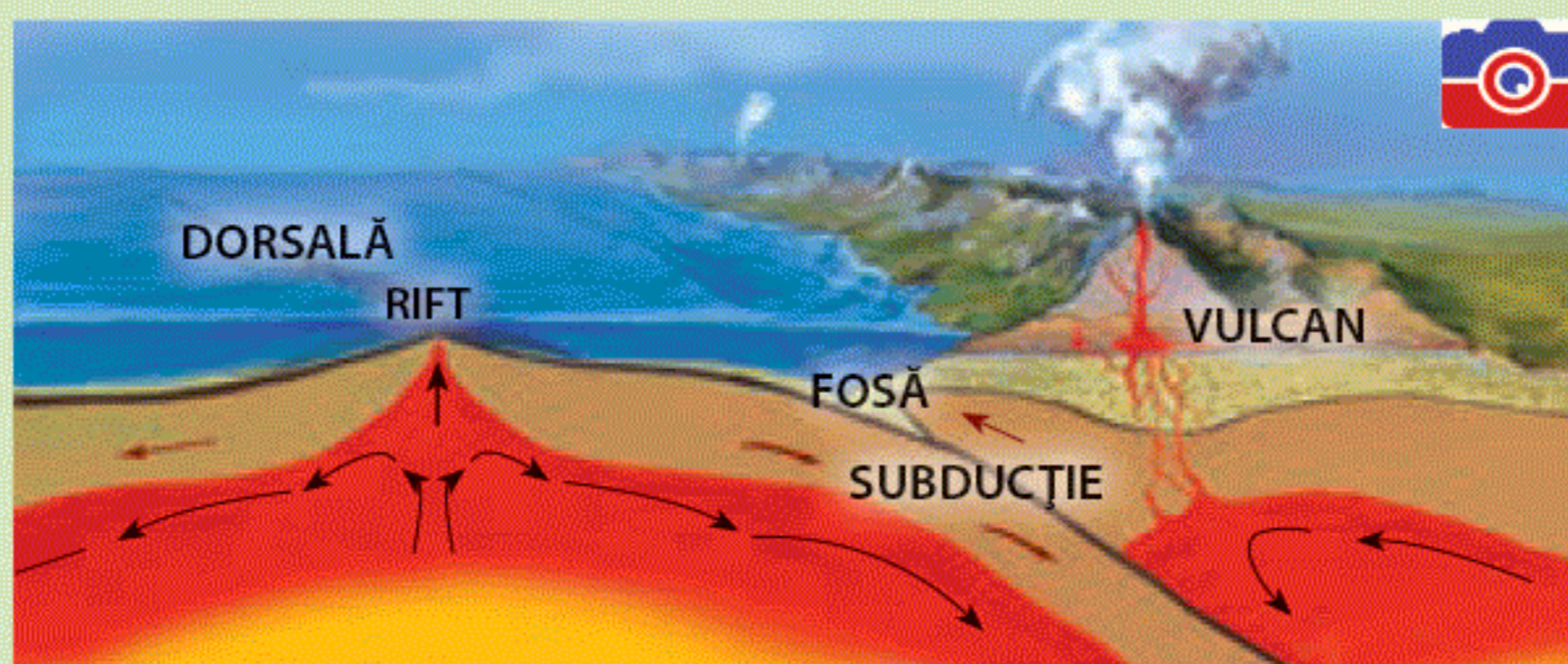
Fig. 1. Rift și subducție
