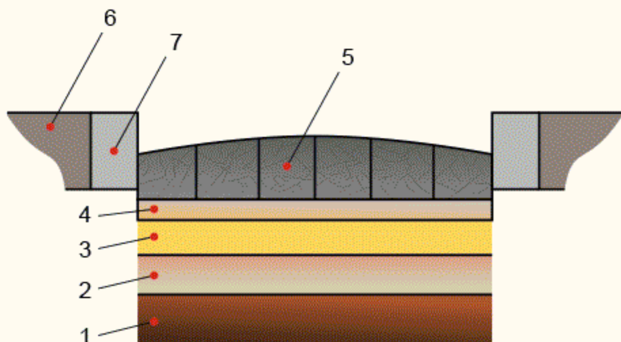
Fig. 2. Secțiune a unui drum roman din orașul Pompei: 1. Pământ; 2. Pietre de mici dimensiuni; 3. Moloz compus din piatră și var; 4. Placă de ciment (cioburi de ceramică pisate și var); 5. Partea superioară a drumului alcătuită din piatră; 6. Trotuar; 7. Borduri.
